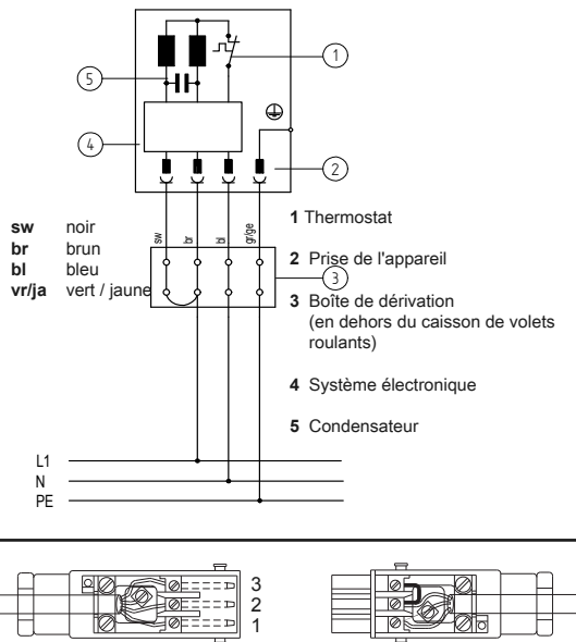
Fig. 5: Plan de câblage RolTop-868 230 V / 50 Hz et pose du câble avec raccord enfichable Hirschmann STAS-3 (avec pont)
