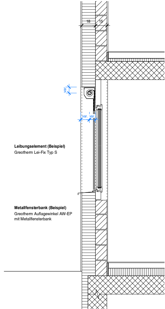
Querschnitt
