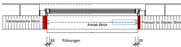
Grundriss
