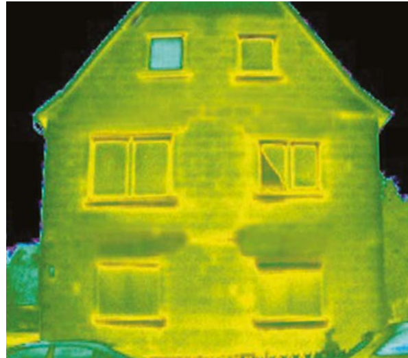
Rollladenkästen sind isoliert. Die Kältebrücke ist geschlossen.
